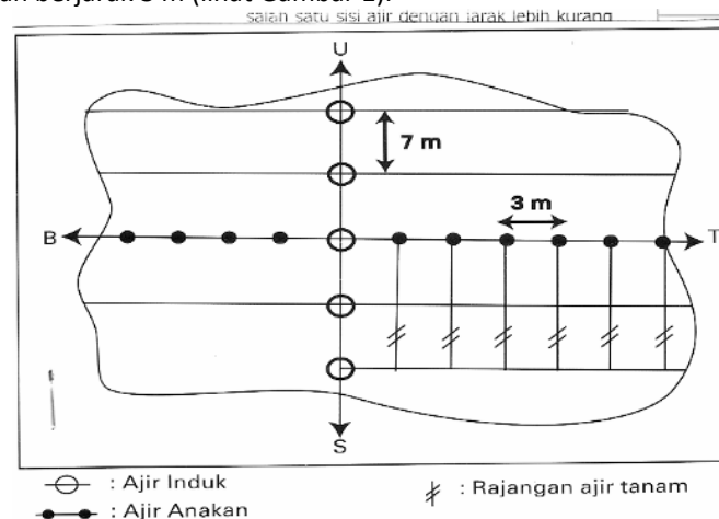
Gambar 1. Cara Pengajiran pada Lahan Datar
