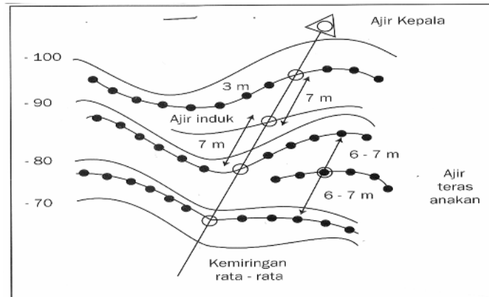
Gambar 2. Cara Pengajiran Menurut Kontur.
